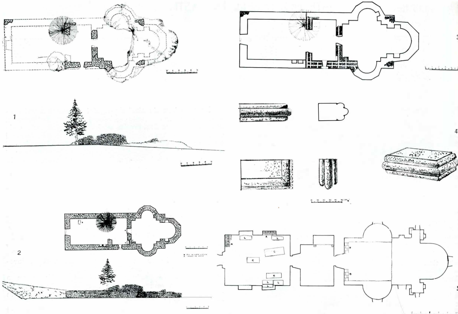
Fig. 1. Plan și elevație înainte de restaurare. Fig. 2. Plan și elevație după restaurare. Fig. 3. Planul canalelor în zid (detaliu). Fig. 4. Bloc de piatră profilat. Fig. 5. Planul pardoselii.
